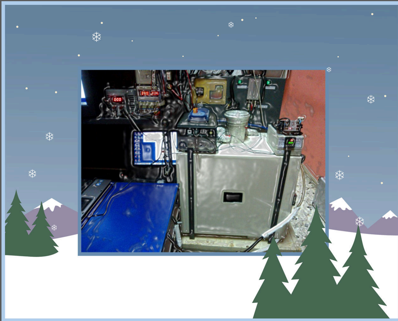
Controllo di pressione e temperatura in box di sicurezza
